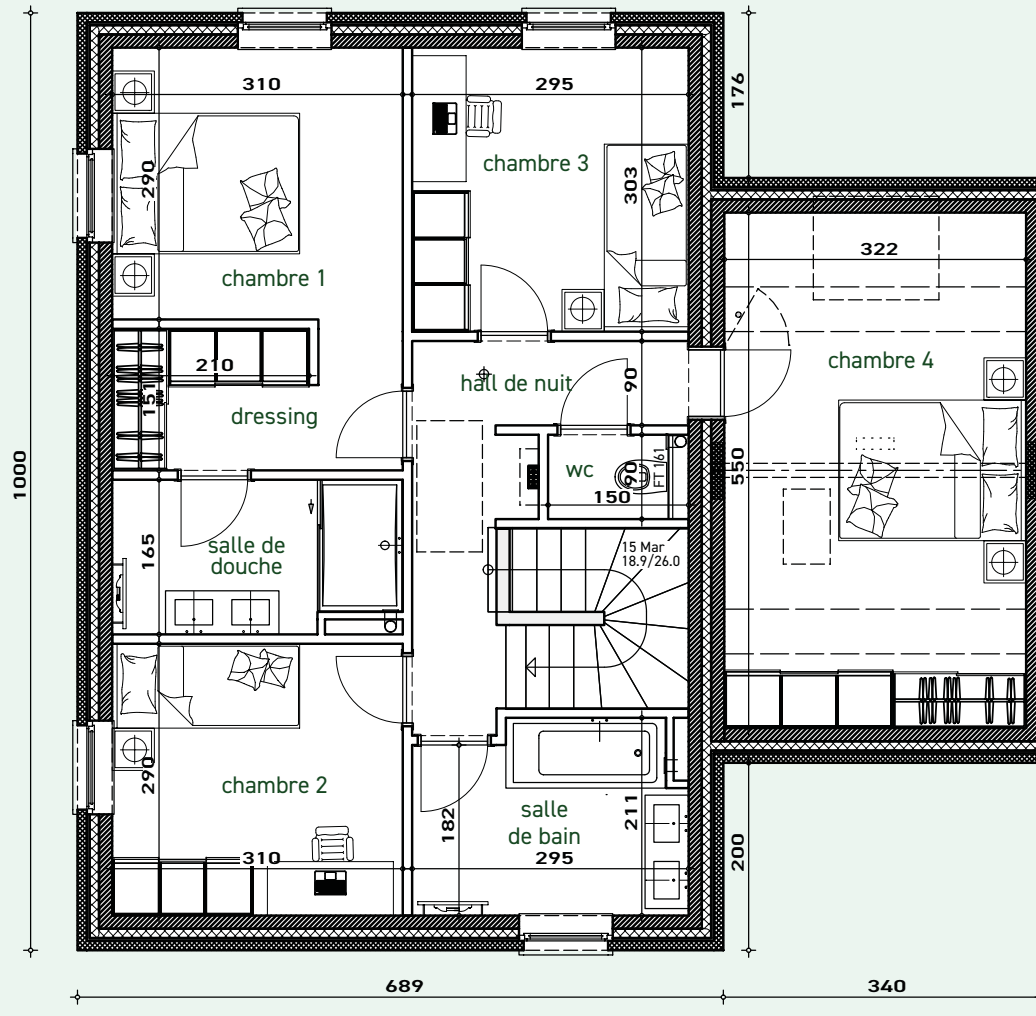
Étage: 90,12 m 2
