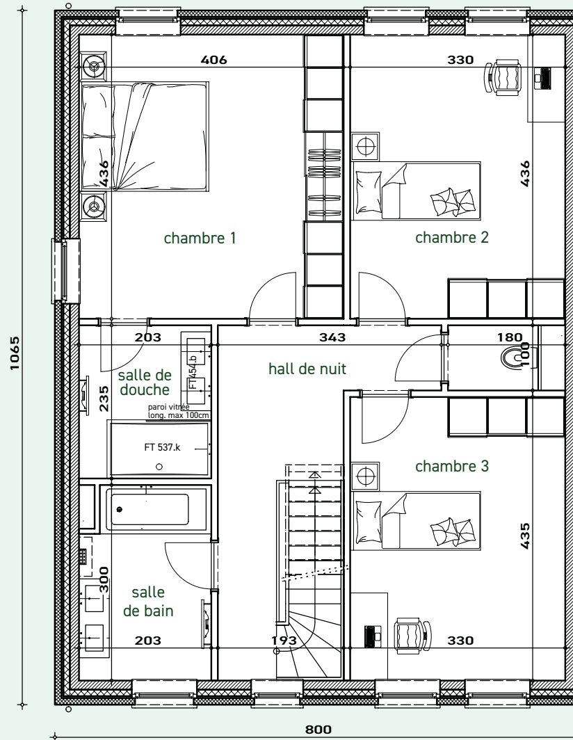
Étage: 85,20 m 2
